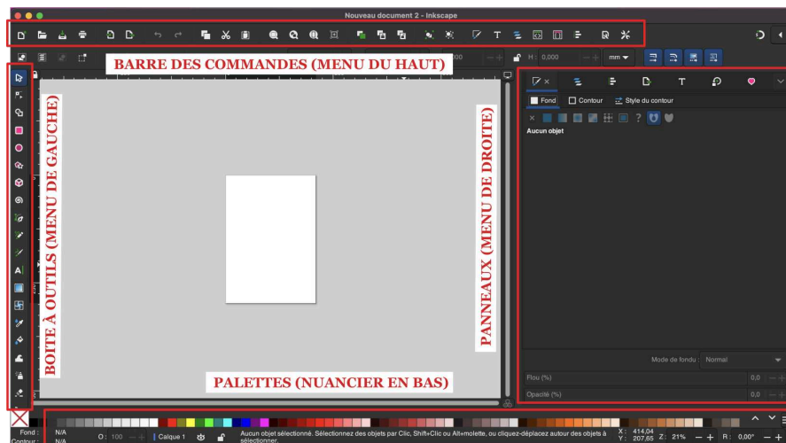
Figure 4.1 : L'interface d'Inkscape
